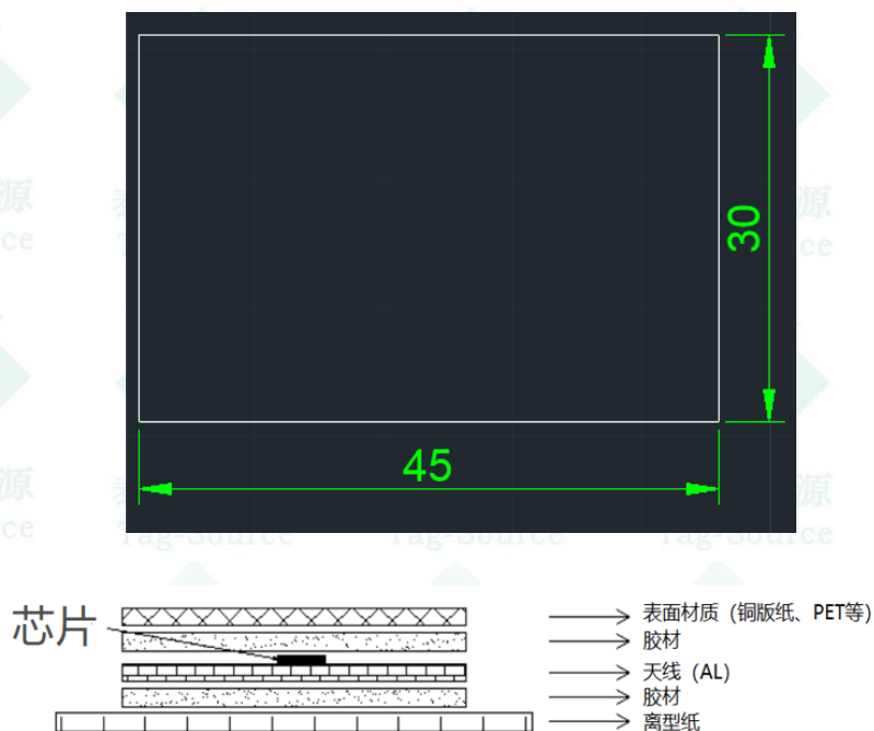
标签结构示意图
