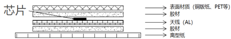
标签结构示意图
